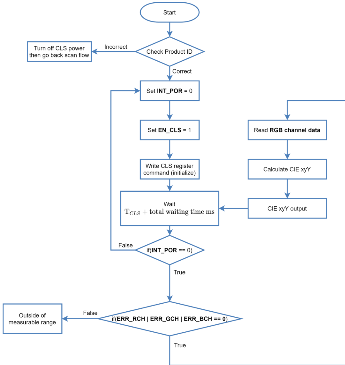
图 8. Firmware 流程图
