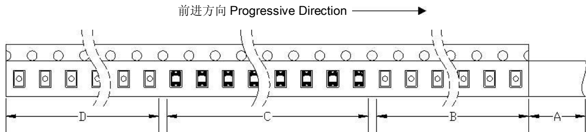
A: 盖带, 300 mm; B: 引导, 空带, 200mm; C: 编载产品 3000只; D: 尾部, 空带, 200mm A: Top Cover Tape, 300mm; B: Leader, Empty, 200mm; C: 3000 Lamps Loaded; D: Trailer, Empty, 200mm.
